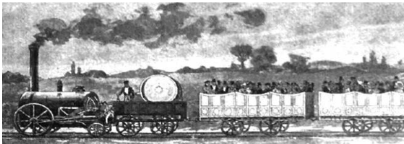
72. Қаторои Манчестер-Ливерпул
