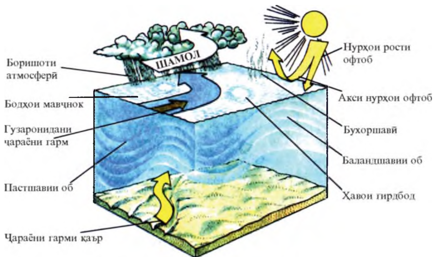
Расми 16. Алюкамандии уқёнус бо атмосфера
