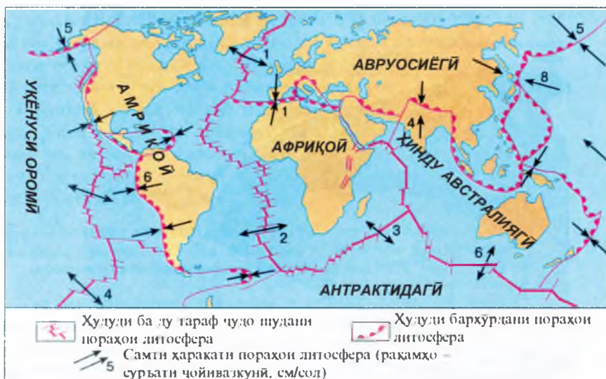
Расми 8. Пораҳои литосфера
