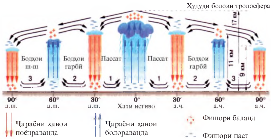
Расми 11. Нақшаи ҳаракати ҳаво дар тропосфера
