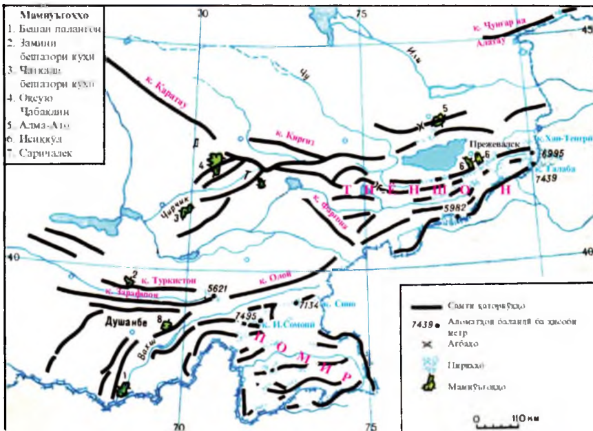
Расми 80. Нақшаи ҷойгиршавии қаторқўҳҳои Тиёншон ва Помир
