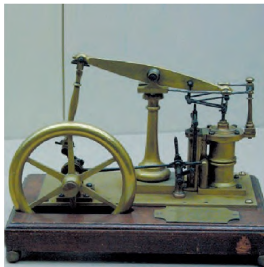
Ուատոնի շոգեմեքենայի մոդելը
