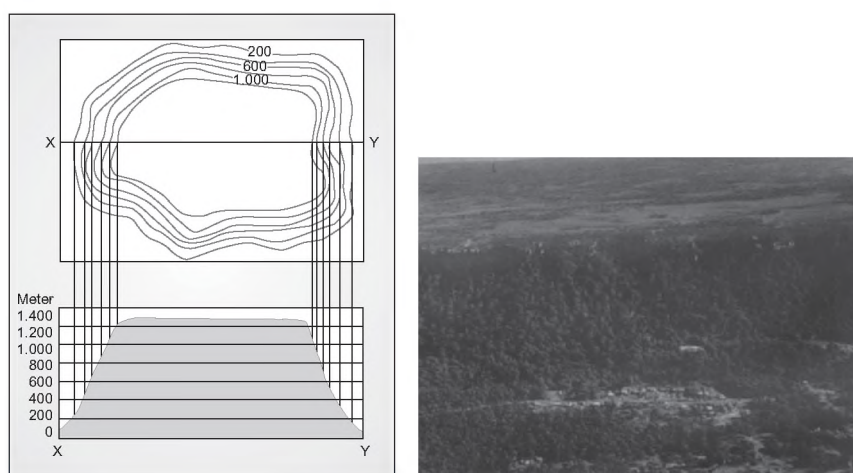
Gambar 5.7 Kontur dan penampang melintang plato serta kenampakan aslinya.
