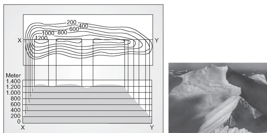
Gambar 5.8 Kontur dan penampang melintang ridge serta kenampakan aslinya.
