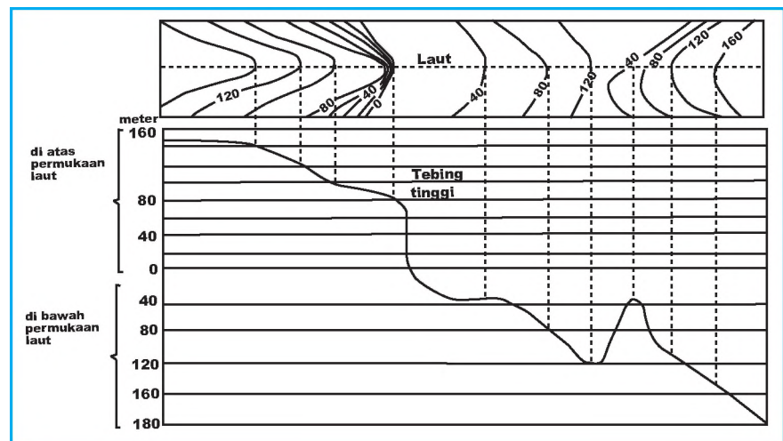
Ilustrasi: Puguh Supriyanto Gambar 5.11 Penampang melintang relief dasar laut.
