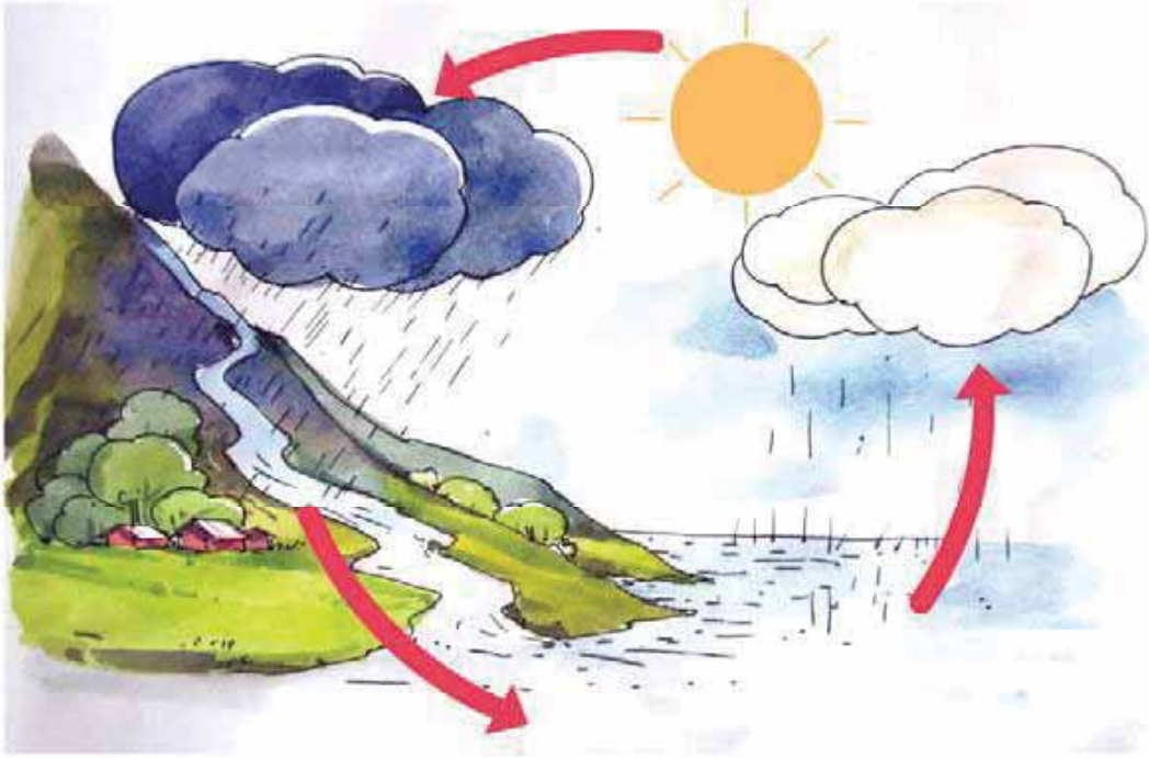
চিত্র: পানিচক্র
