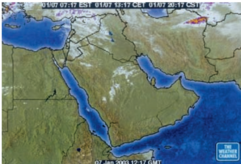
شکل ۹- نمونه‌ای از نقشه‌ی هواشناسی تهیه شده از ماهواره‌ی نوآ — منطقه‌ی خاور میانه
