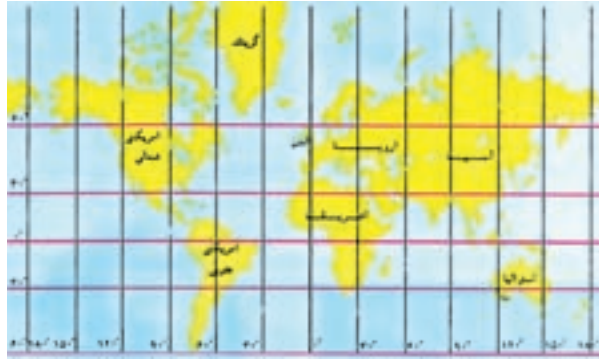
شکل ۷ — سیستم تصویر استوانه‌ای
