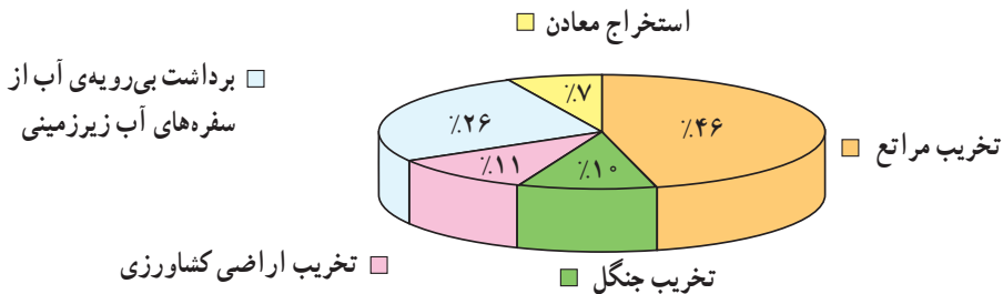
شکل ۲- نمودار درصد سهم عوامل مختلف در روند بیابان‌زایی در ایران
